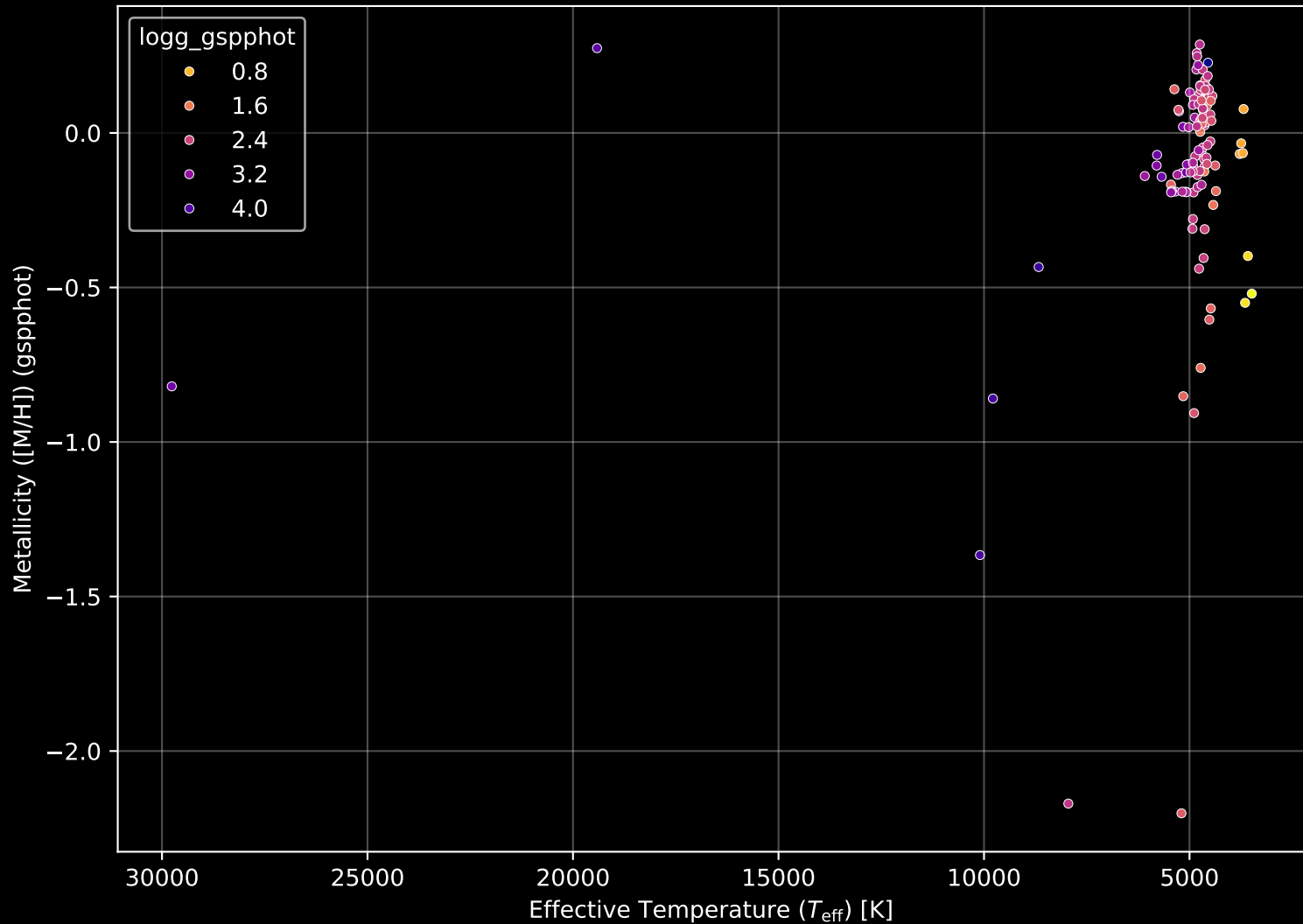
APOGEE DR17 Field: [COL261] Stellar Population Parameters (n= 117)
